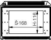
Pohled zespodu
