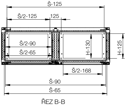
Řez, pohled shora (bez spodní desky)
