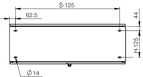
Řez, pohled shora (bez spodní desky)
