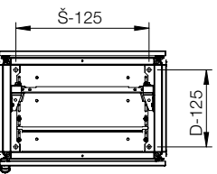
Řez, pohled shora
