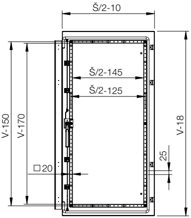
Levé dveře, pohled zevnitř
