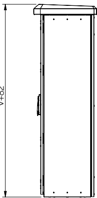
Dešťová clona, pohled z boku
