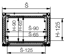
ŘEZ A-A
