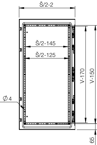
Pravé dveře, pohled zevnitř
