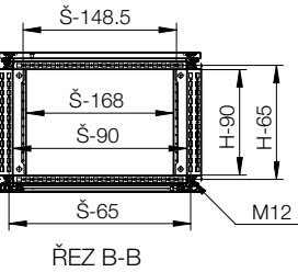
Řez, pohled shora (bez spodní desky)
